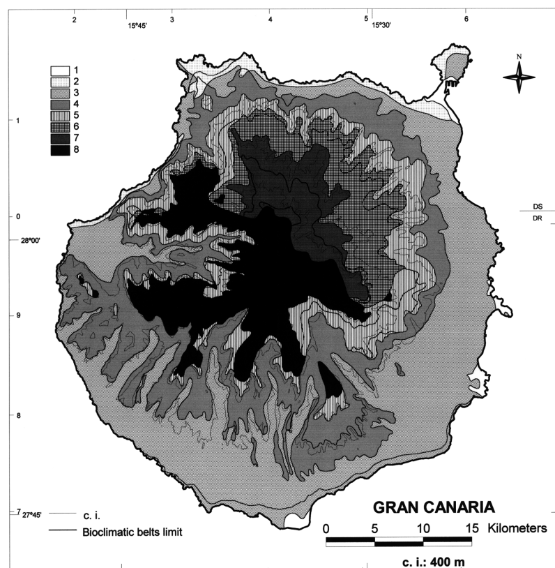
Fig. 8. Map of potential natural vegetation. — 1: Edaphophilous sabulicolous inframediterranean Western Canary geosigmetum . — 2: Astydiamio-Euphorbio aphyllae sigmetum ; — 3: Euphorbio balsamiferae sigmetum ; — 4: Aeonio percarnei-Euphorbio canariensis sigmetum ; — 5: Pistacio lentisci-Oleo cerasiformis sigmetum ; — 6: Visneo mocanerae-Arbuto canariensis sigmetum ; — 7: Lauro azoricae-Perseo indicae sigmetum ; — 8: Pino canariensis sigmetum .
